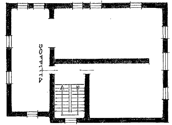
SECONDO PIANO H=2.80
