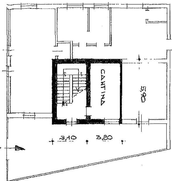
PIANO TERRA H=3.30
